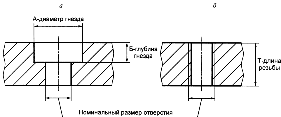
a — без резьбы; b — с резьбой
